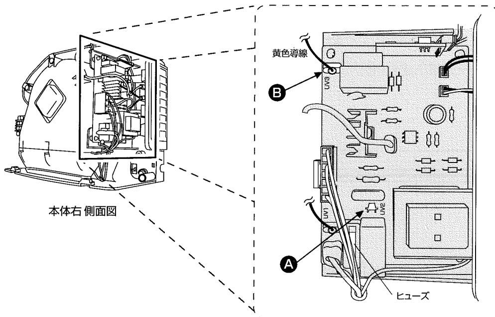
図1 (メイン基板の拡大図)
