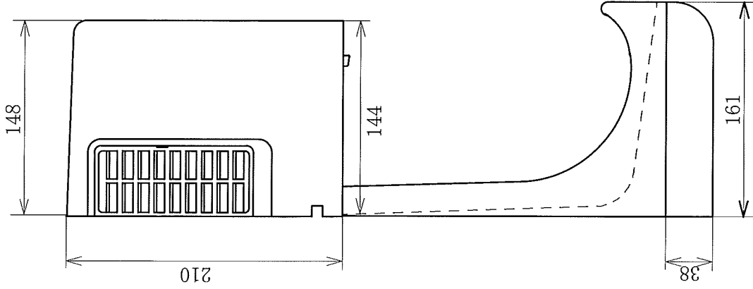
側面図
