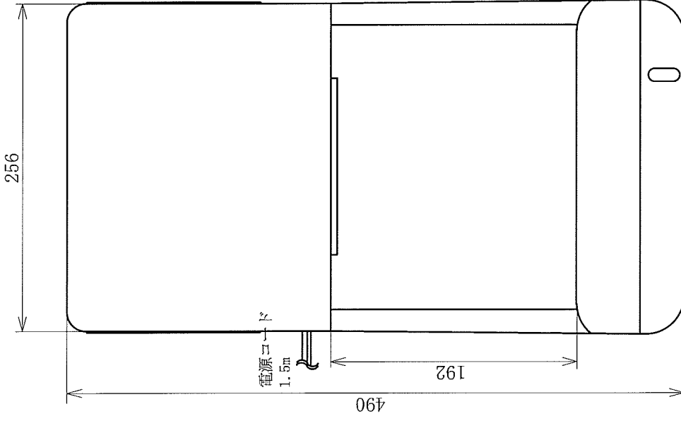
正面図
