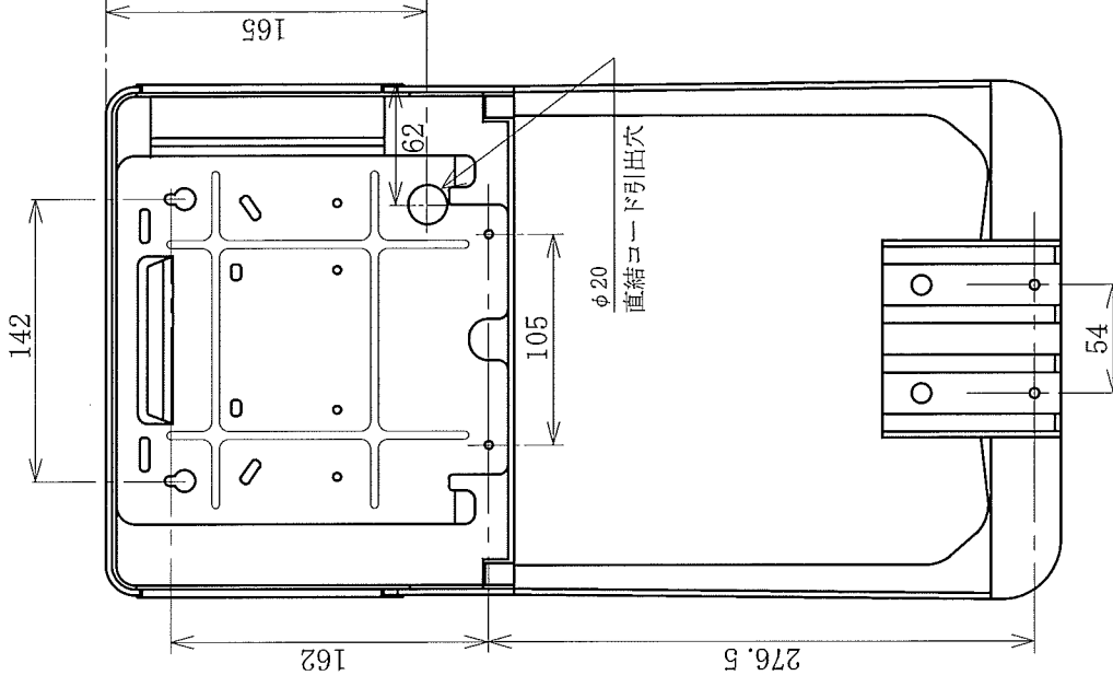
背面図
