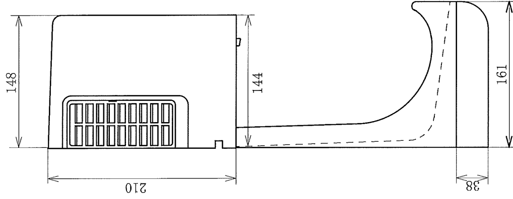
側面図
